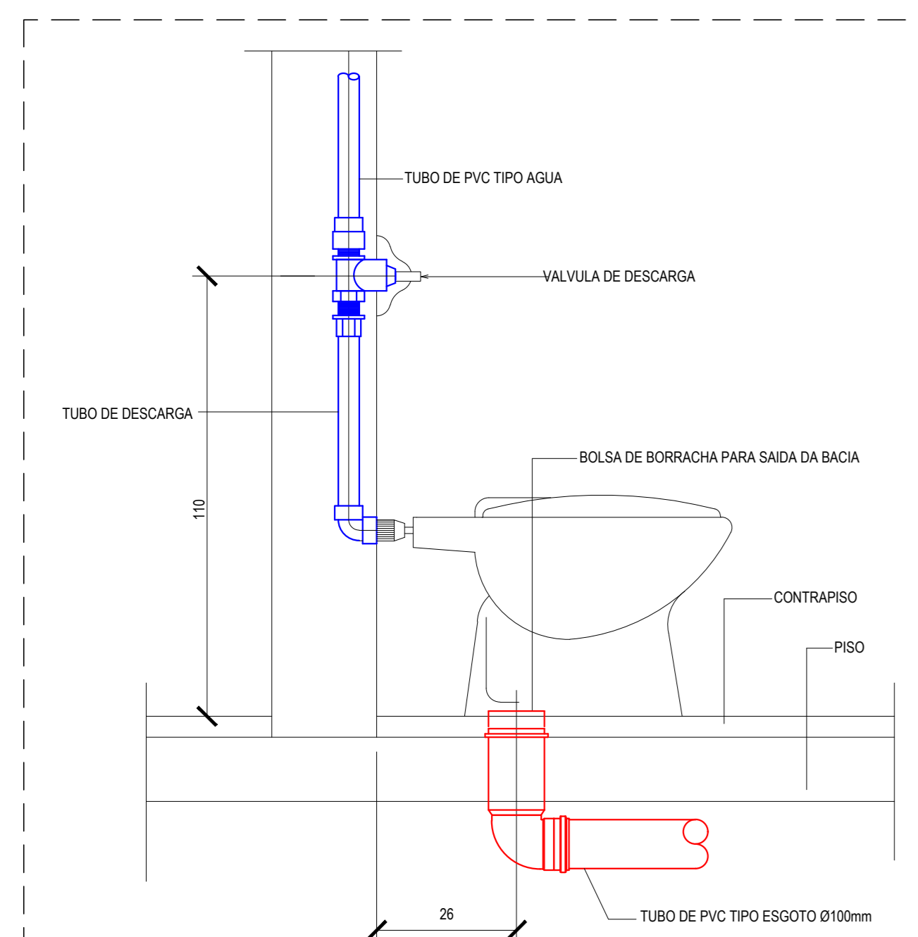
DETALHE VASO SEM ESCALA
