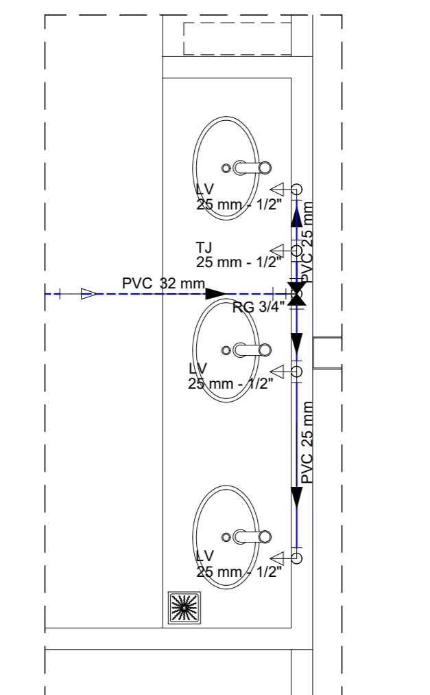
DETALHE - H2 ESCALA 1:25
