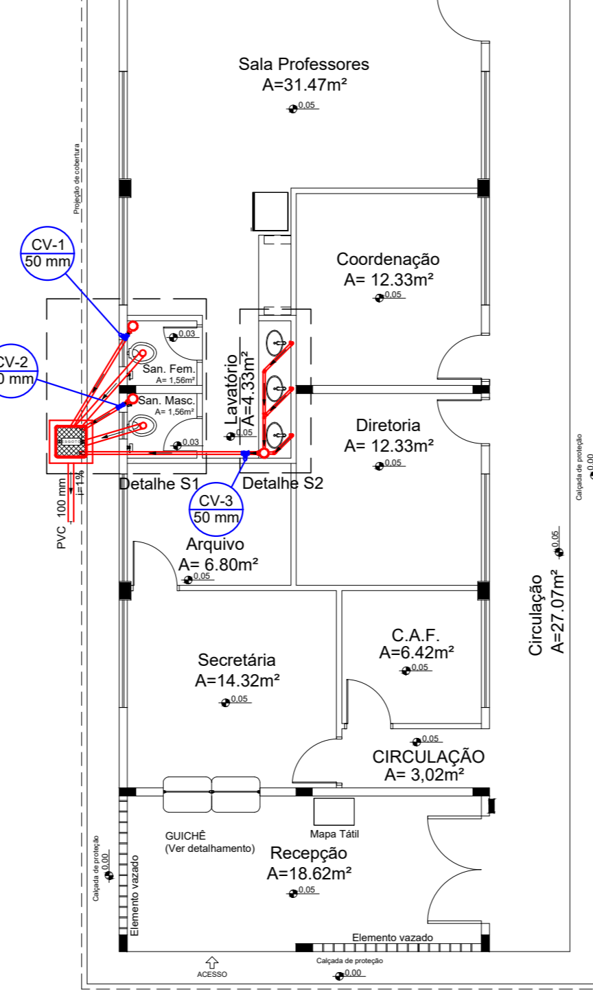
PLANTA - ESG. TÉRREO ESCALA 1:100
