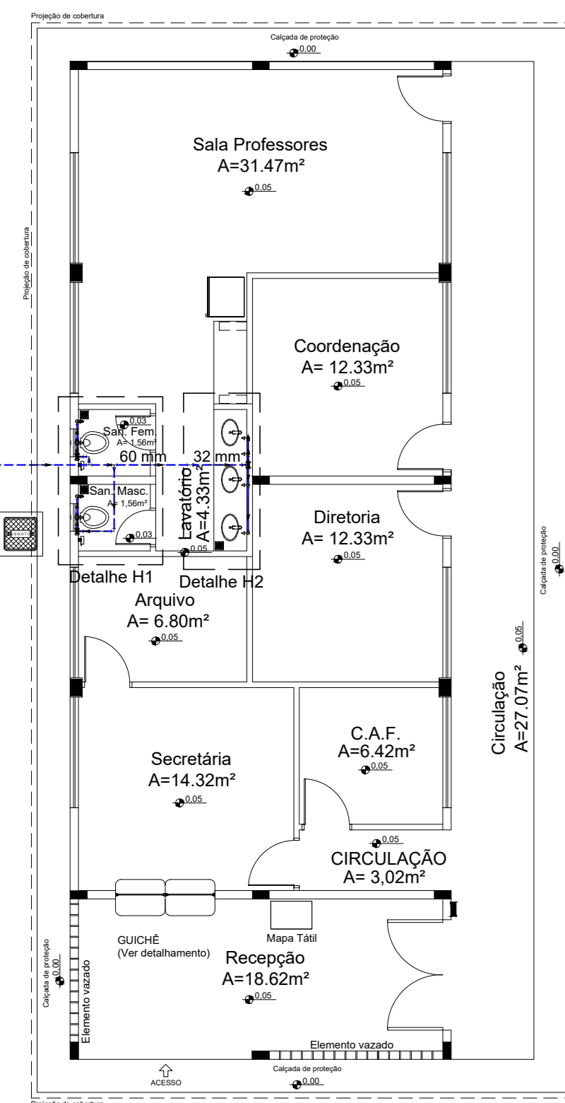
PLANTA - HID. TÉRREO ESCALA 1:100
