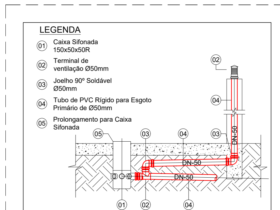
DETALHE VENTILAÇÃO SEM ESCALA
